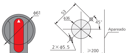
Gráfico de perforación del montaje de la palanca
